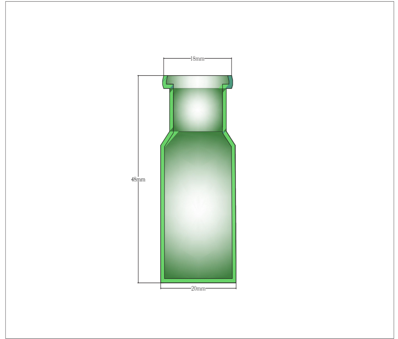
SECTION 1:1
